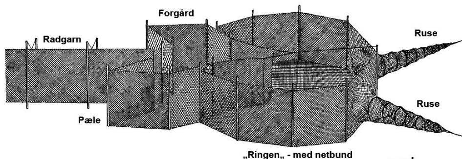
Ruse Type 4 - det egentlige bundgarn med flere samleruser koblet på selve „ringen„ (flere overgangsformer forekommer ofte)
